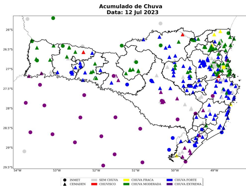
Figura 7: Acumulado diário de precipitação sobre o estado de Santa Catarina para o dia 12 de julho, baseados nas estações meteorológicas do INMET e CEMADEN
