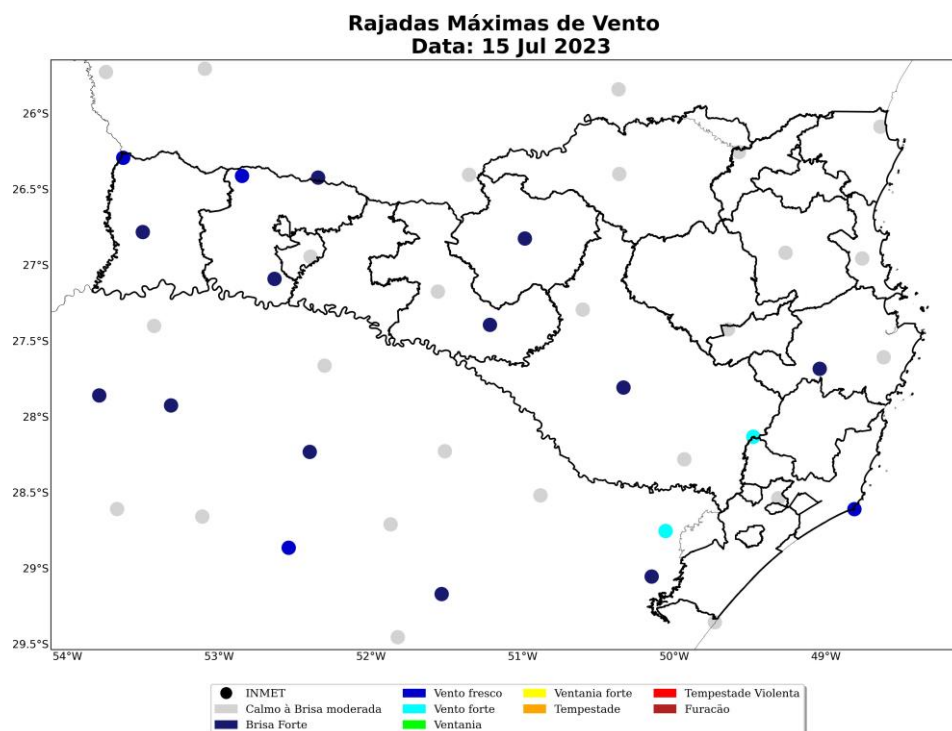
Figura 15: Rajada de vento sobre o estado de Santa Catarina para o dia 15 de julho, baseado nas estações meteorológicas do INMET
