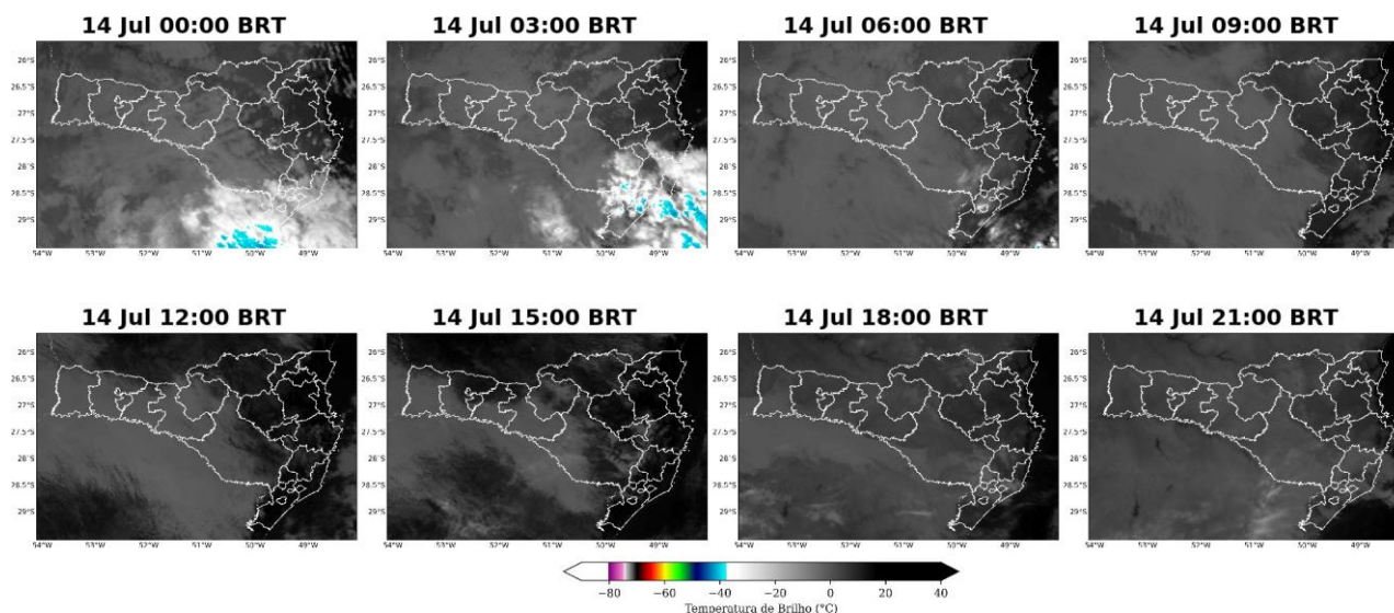
Figura 4: Imagens realçadas do satélite GOES-16 das 00 BRT até 21 BRT (a cada 3 horas) para o dia 14 de julho.
