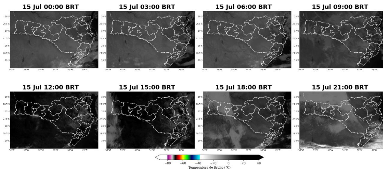
Figura 5: Imagens realçadas do satélite GOES-16 das 00 BRT até 21 BRT (a cada 3 horas) para o dia 15 de julho.
