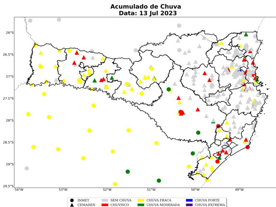
Figura 8: Acumulado diário de precipitação sobre o estado de Santa Catarina para o dia 13 de julho, baseados nas estações meteorológicas do INMET e CEMADEN
