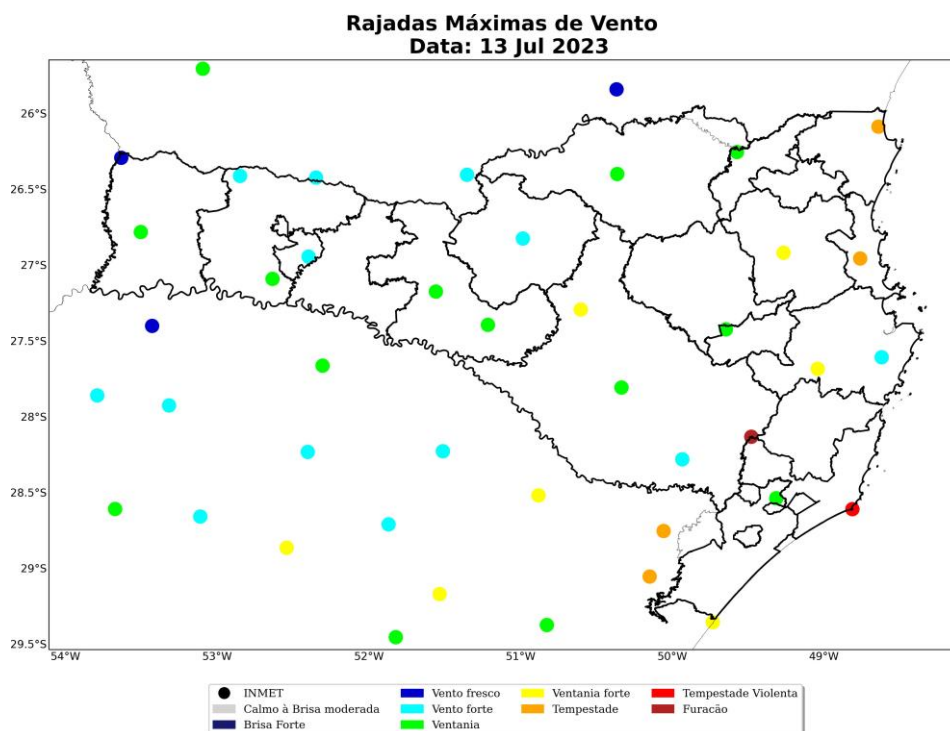
Figura 22: Rajada de vento sobre o estado de Santa Catarina para o dia 13 de julho, baseado nas estações meteorológicas do INMET
