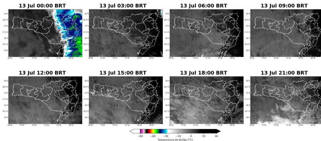
Figura 3: Imagens realçadas do satélite GOES-16 das 00 BRT até 21 BRT (a cada 3 horas) para o dia 13 de julho.
