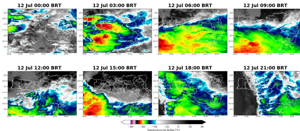
Figura 2: Imagens realçadas do satélite GOES-16 das 00 BRT até 21 BRT (a cada 3 horas) para o dia 12 de julho.
