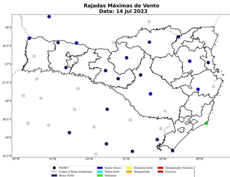
Figura 23: Rajada de vento sobre o estado de Santa Catarina para o dia 14 de julho, baseado nas estações meteorológicas do INMET
