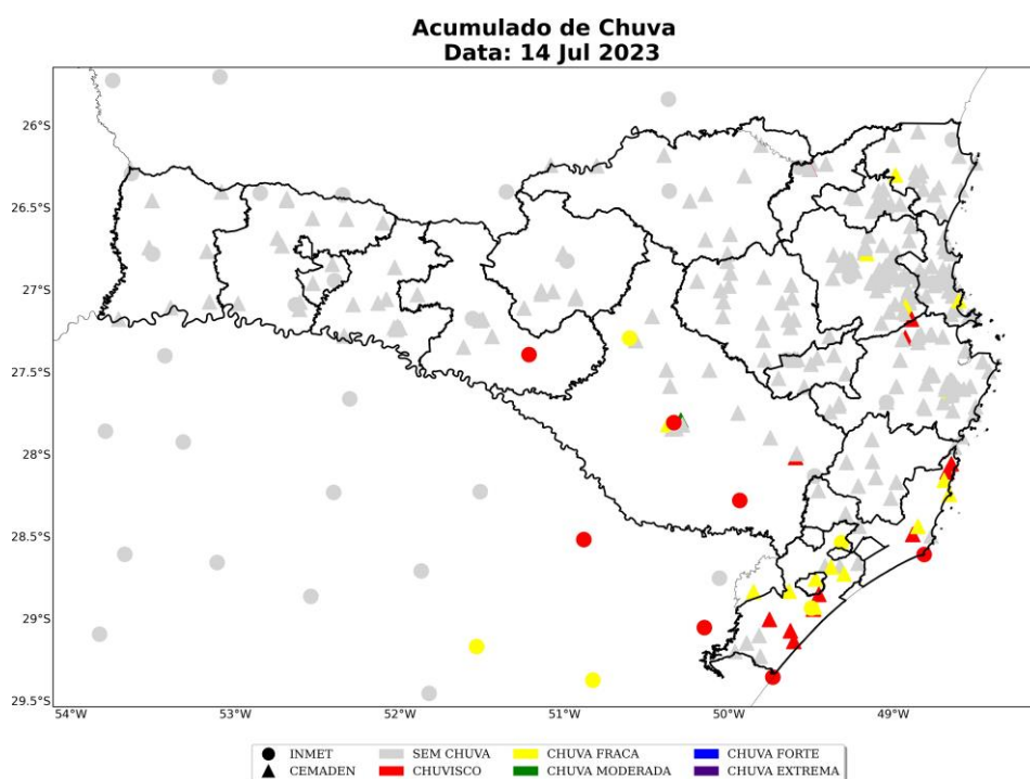
Figura 9: Acumulado diário de precipitação sobre o estado de Santa Catarina para o dia 14 de julho, baseados nas estações meteorológicas do INMET e CEMADEN
