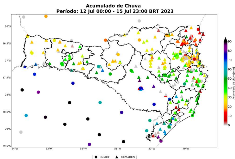
Figura 11: Acumulado diário de precipitação sobre o estado de Santa Catarina para o período de 12 a 15 de julho de 2023, baseado nas estações meteorológicas do INMET e CEMADEN
