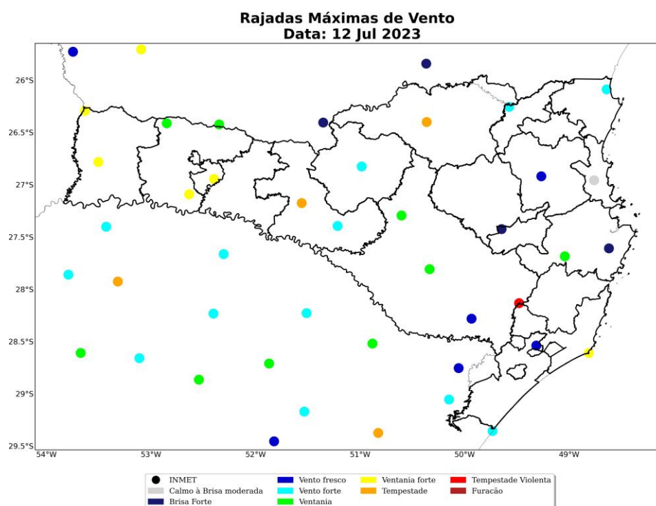
Figura 212: Rajada de vento sobre o estado de Santa Catarina para o dia 12 de julho, baseado nas estações meteorológicas do INMET
