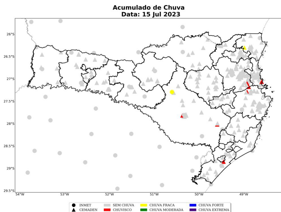
Figura 10: Acumulado diário de precipitação sobre o estado de Santa Catarina para o dia 15 de julho, baseados nas estações meteorológicas do INMET e CEMADEN
