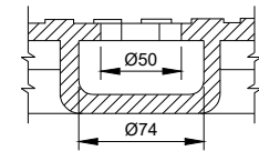
CORTE - CC'
