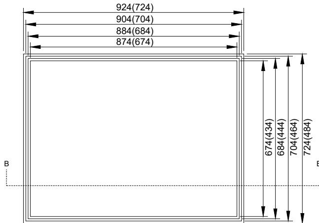
ARO PARA A TAMPA DA CAIXA DE PASSAGEM
