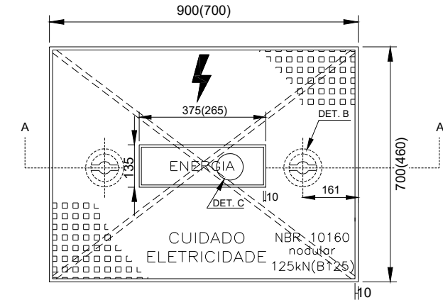
TAMPA DA CAIXA DE PASSAGEM 900x700 [B1] ou (700x460) [A1]
