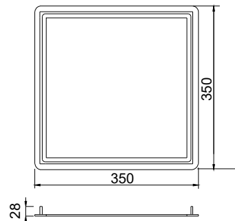
ARO DA TAMPA DA CAIXA DE INSPEÇÃO DE ATERRAMENTO
