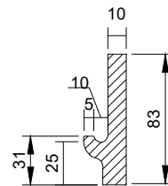
DETALHE - D
