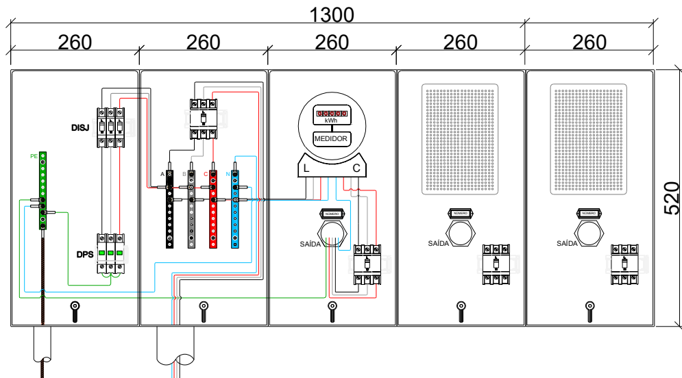
VISTA FRONTAL TAMPA DISJUNTOR GERAL
