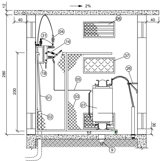
CORTE A-A'
