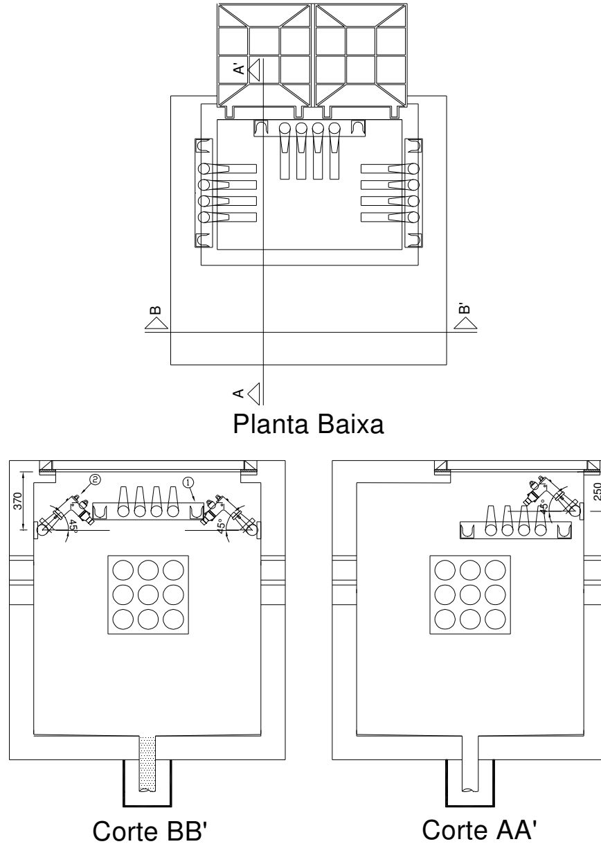
Figura 40 – Instalação de BTX e BQX em caixas E
