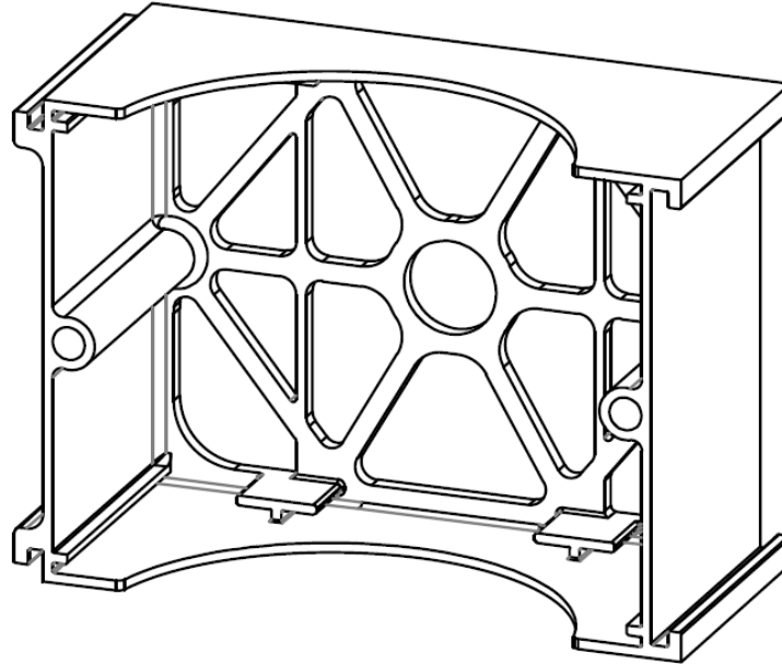
Figura 24 – Espaçador Modular para Banco de dutos - Código Celesc 43347
