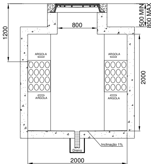
Corte AA'
