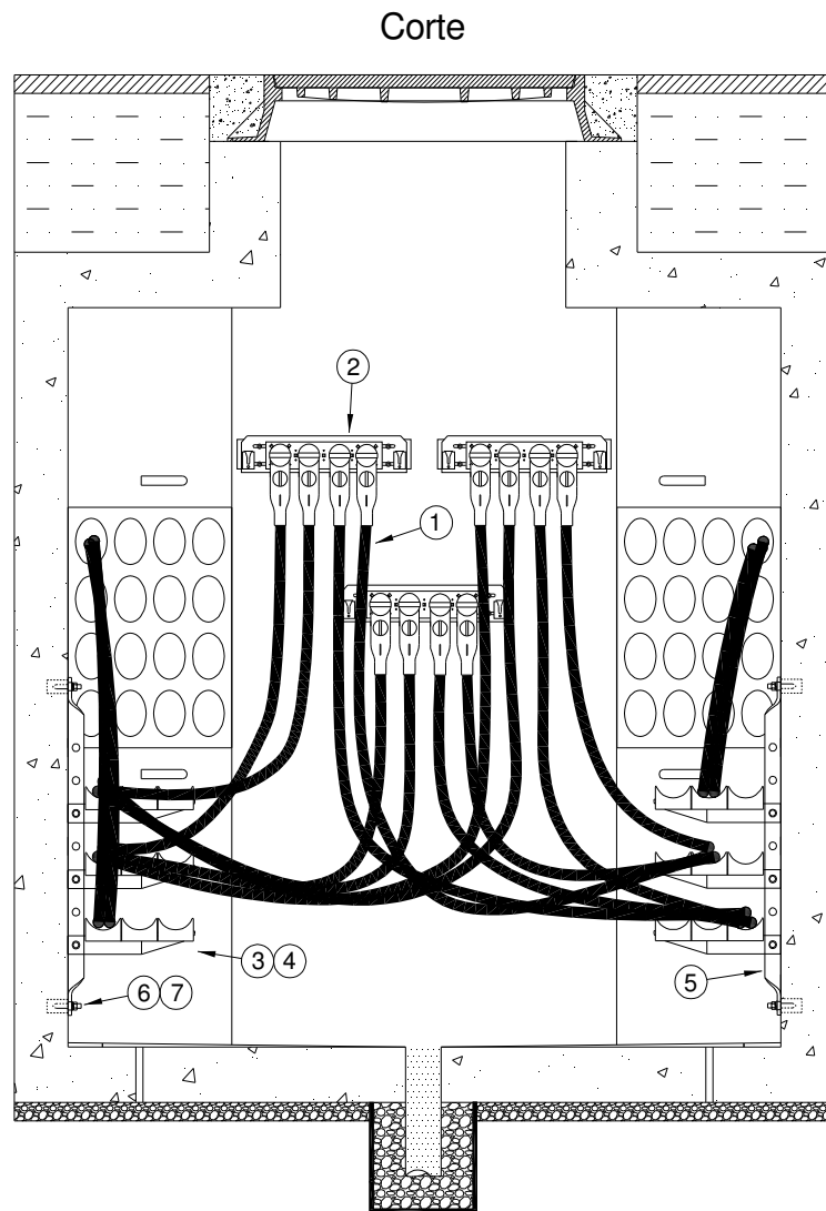
Figura 45 – Exemplo de Montagens de Desconectáveis 200 A em Caixas tipo M (BTX ou BQX)
