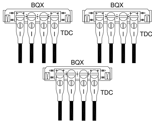
Figura 45 – Exemplo de Montagens de Desconectáveis 200 A em Caixas tipo M (BTX ou BQX)
