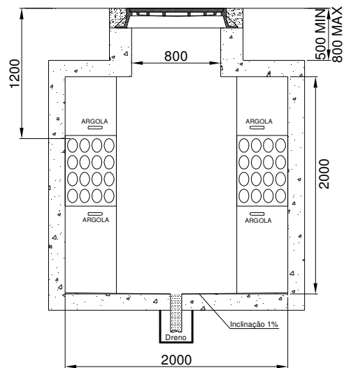
Corte BB'
