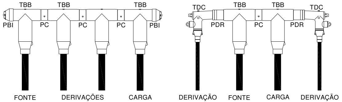
Figura 47 – Montagens de Desconectáveis 600 A em Caixas tipo M (Duas Derivações)
