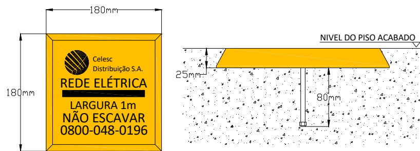
Figura 3 - Placa de Identificação de Traçado de Rede Elétrica Subterrânea
