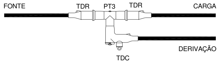
ESQUEMA DE MONTAGEM
