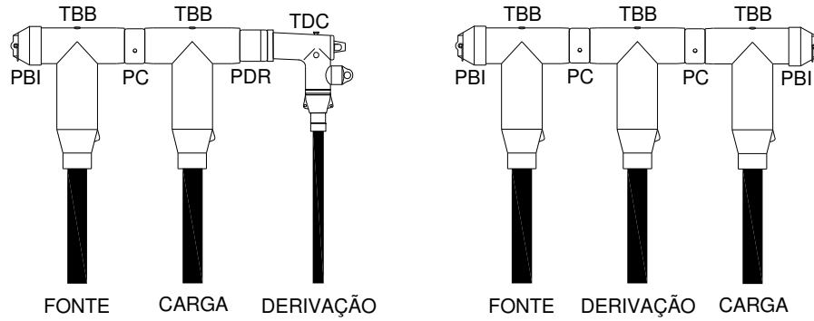
Figura 46 – Montagens de Desconectáveis 600 A em Caixas tipo M (Uma Derivação)
