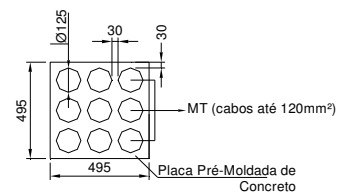
Placa Entrada/Saída Dutos
