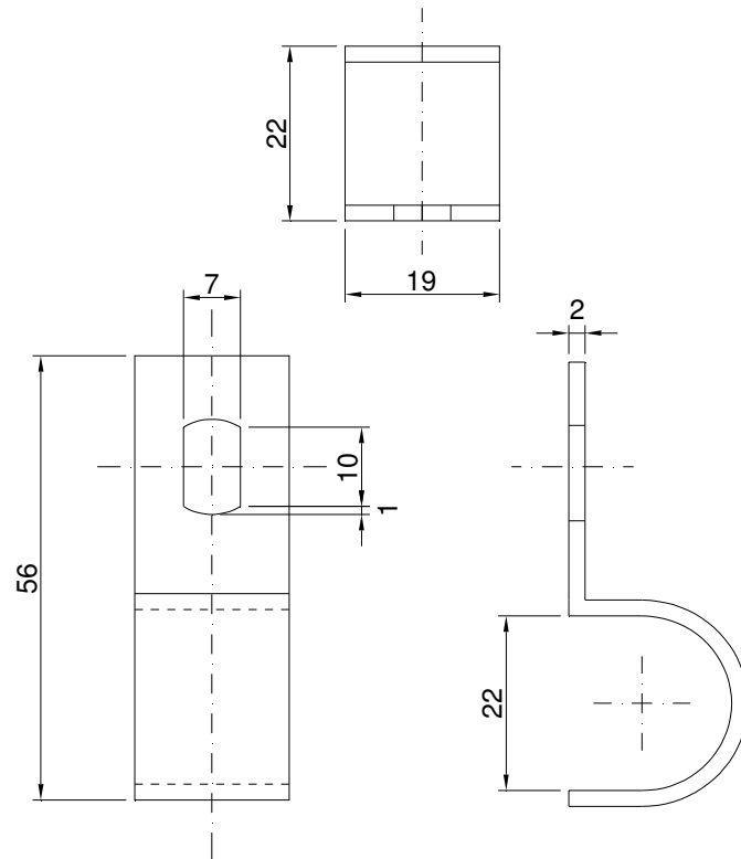
Figura 28 – Abraçadeira Tipo Unha
