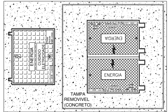
Vista Superior - Tampas
