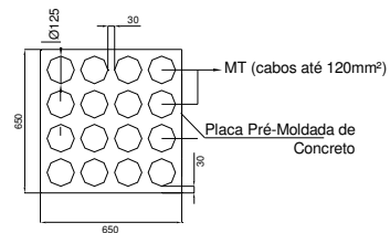
Placa Entrada/Saída Dutos
