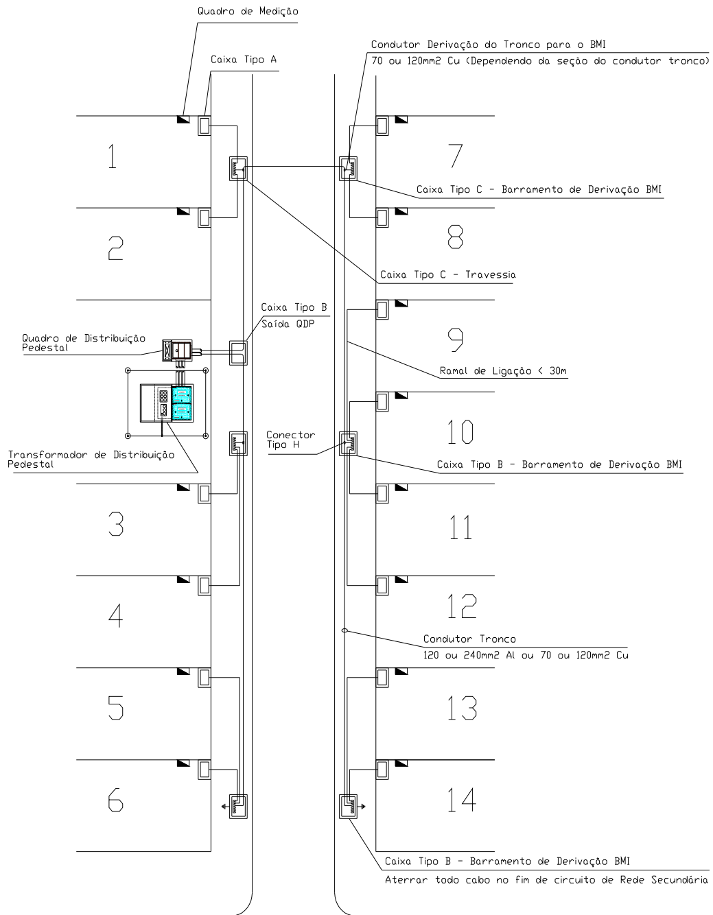
Figura 9 – Concepção Básica de Redes Secundárias
