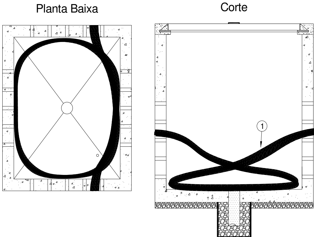
Figura 35 - Instalação de cabo em caixas D e E (sobra de cabo)
