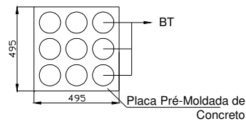
Exemplo Placa Entrada/Saída Dutos
