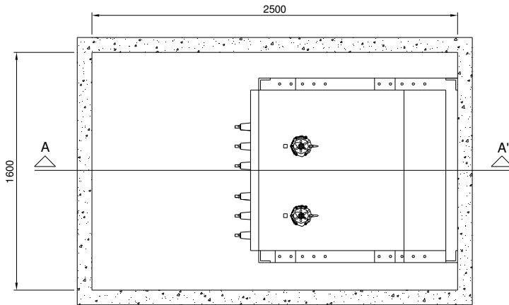
Planta Baixa
