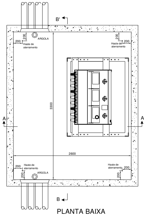
Figura 15 - Caixa CM - Utilizada para instalação de chaves submersíveis (3300x2600x2500mm) - Código Celesc 32684
