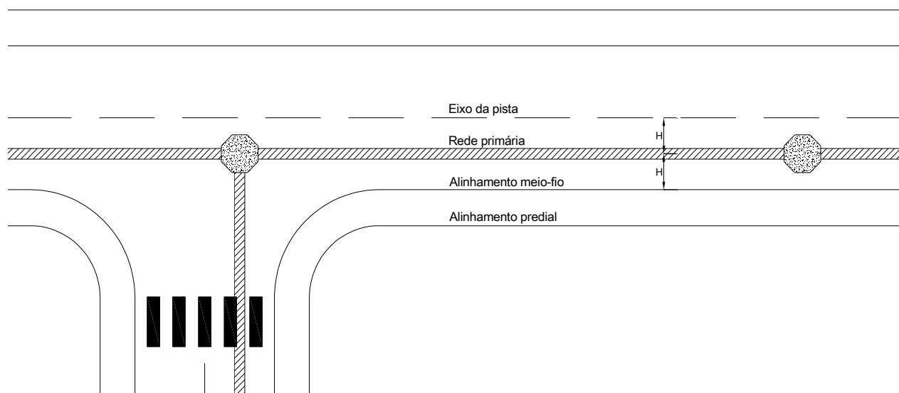
Figura 5 – Traçado de rede de distribuição primária em vias de circulação de veículos
