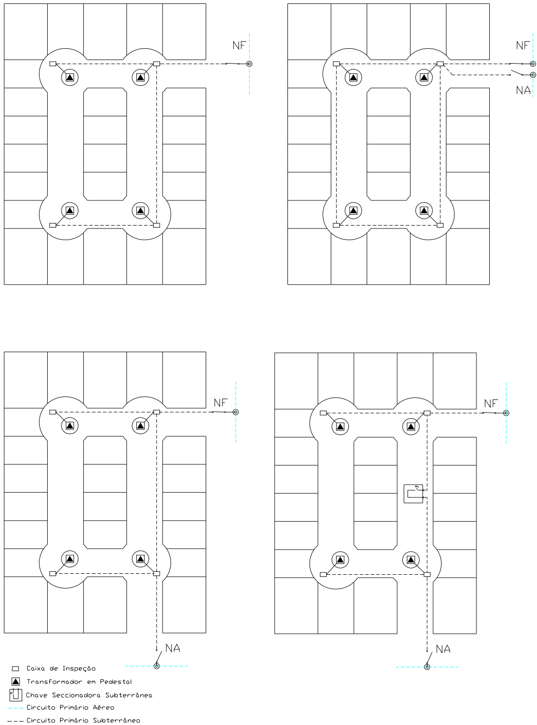
Figura 6 – Exemplos de circuitos primários radiais.
