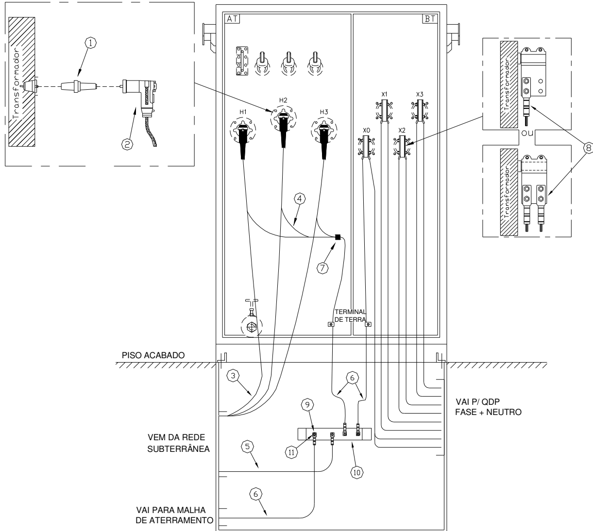
Figura 50 – Conexões dos Transformadores Pedestais
