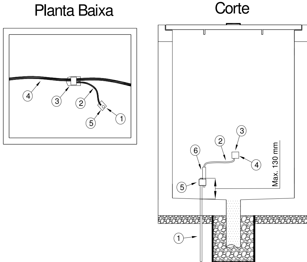
Figura 55 – Instalação de Aterramento em Circuitos de Baixa Tensão
