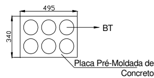
Placa Entrada/Saída Dutos
