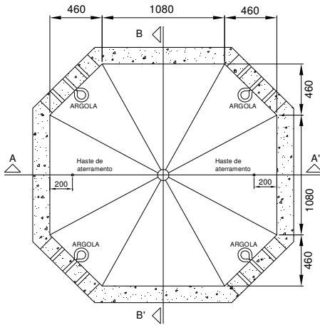
Planta Baixa
