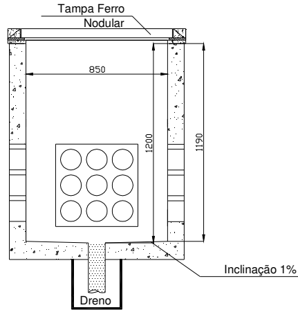
Corte BB'
