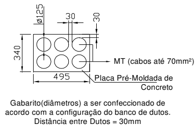
Placa Entrada/Saída Dutos
