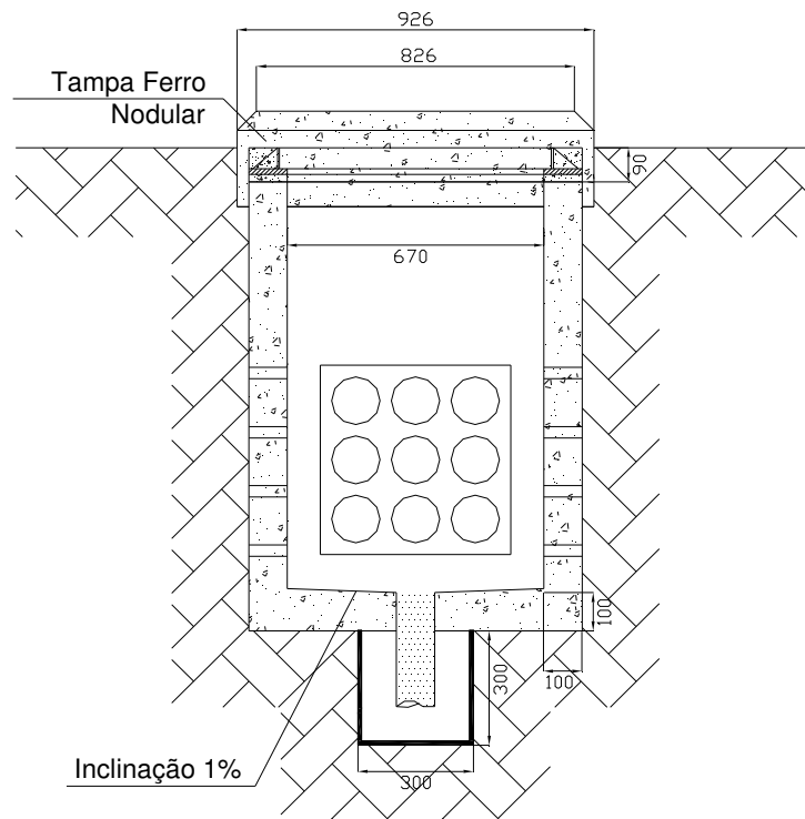
Corte AA
