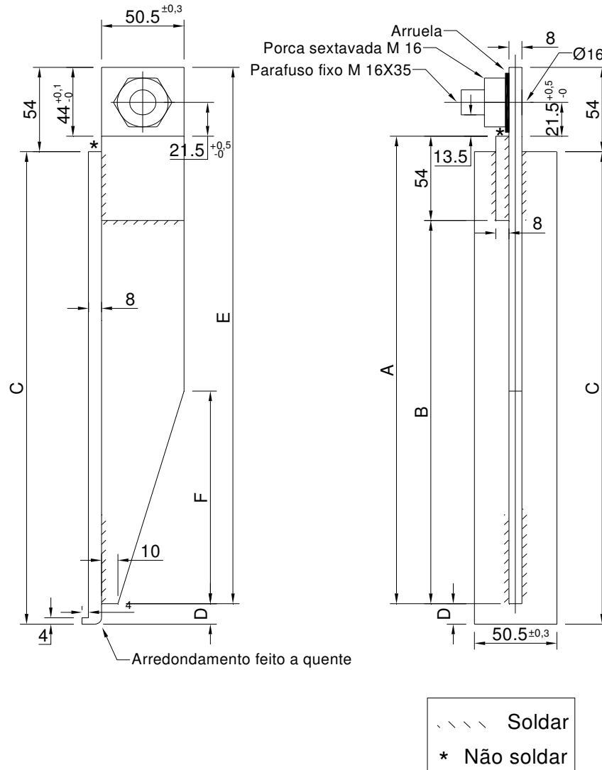
Figura 26 Suporte Horizontal para Apoio de Cabos
