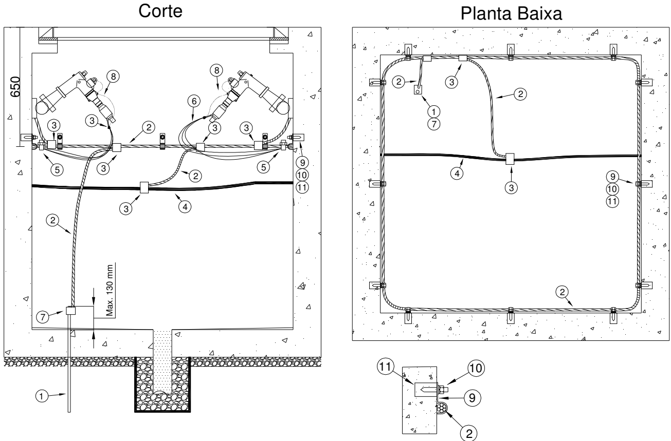
Detalhe da Fixação da Malha
