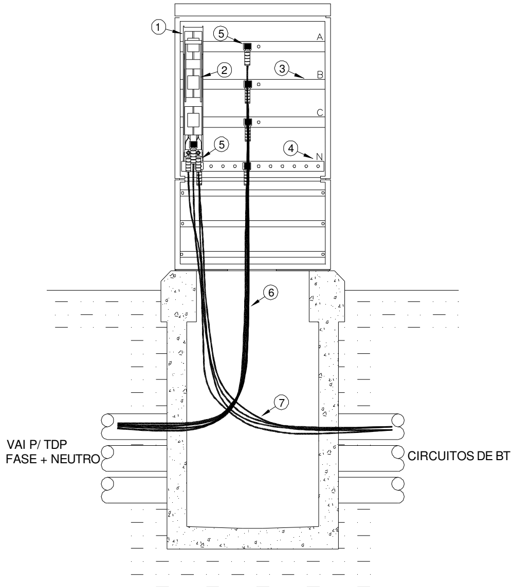
Figura 52 – Conexões Elétricas do Quadros de Distribuição e Proteção
