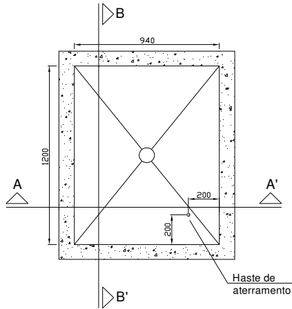
Planta Baixa
