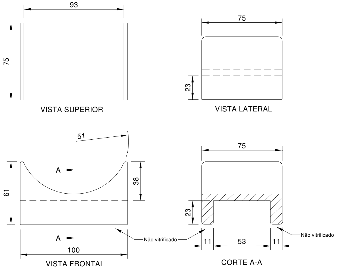
Figura 27 Sela de Porcelana para Apoio de Cabos
