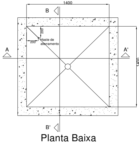
Figura 13 - Caixa E - Utilizada para rede de distribuição primária (MT) para cabos até 120mm 2 , com três linhas de dutos até 9 dutos (1400x1400x1500mm) – Código Celesc 34188
