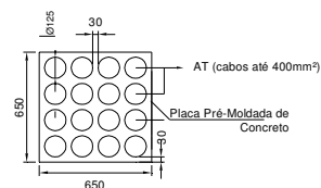
Placa Entrada/Saída Dutos
