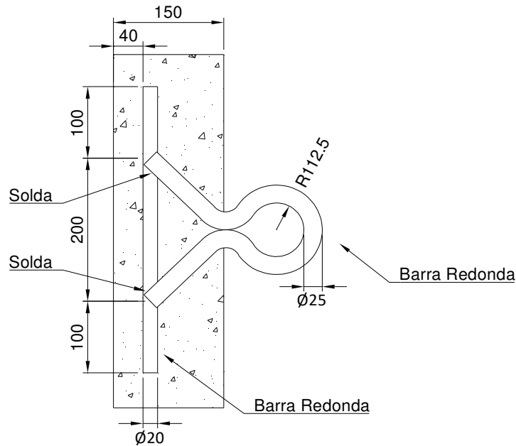
Figura 21 – Argola de puxamento
