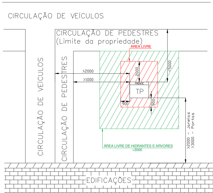
Figura 8 - Instalação de Transformadores - Distâncias Básicas (Dimensões em mm)
