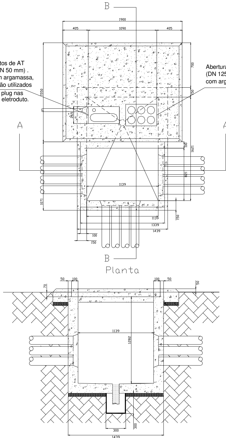
Figura 18 – Base de concreto com caixa acoplada para transformador pedestal - Código Celesc 41310
