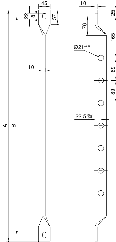
Figura 25 Suporte Vertical para Apoio de Cabos (7 e 15 furos)
