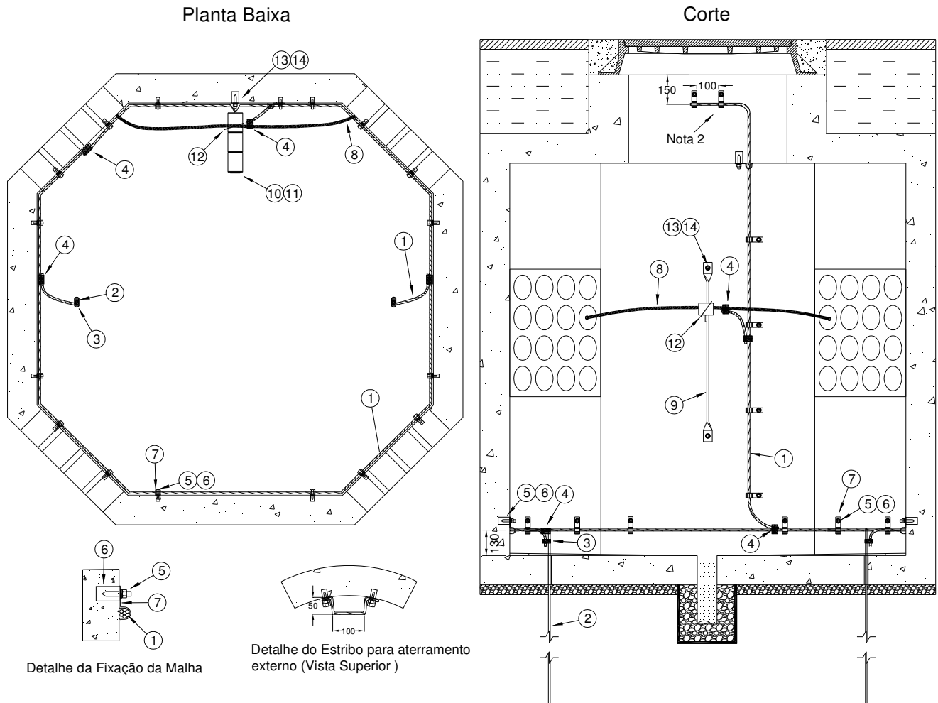
Figura 57 - Instalação de Aterramento e Ligação ao Condutor de Proteção em Caixas Tipo M
