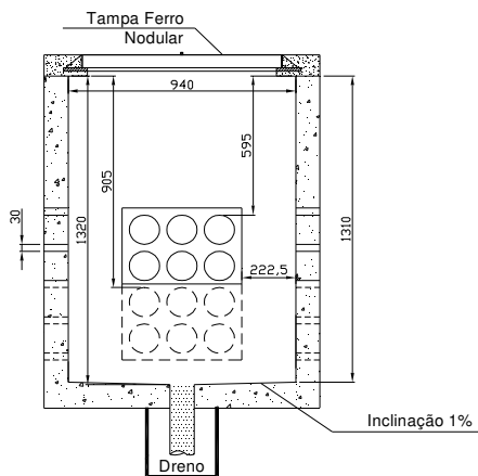
Corte AA'
