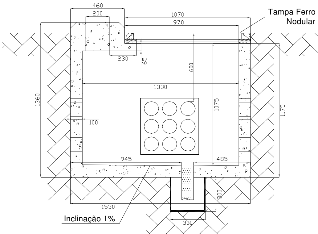
Corte BB
