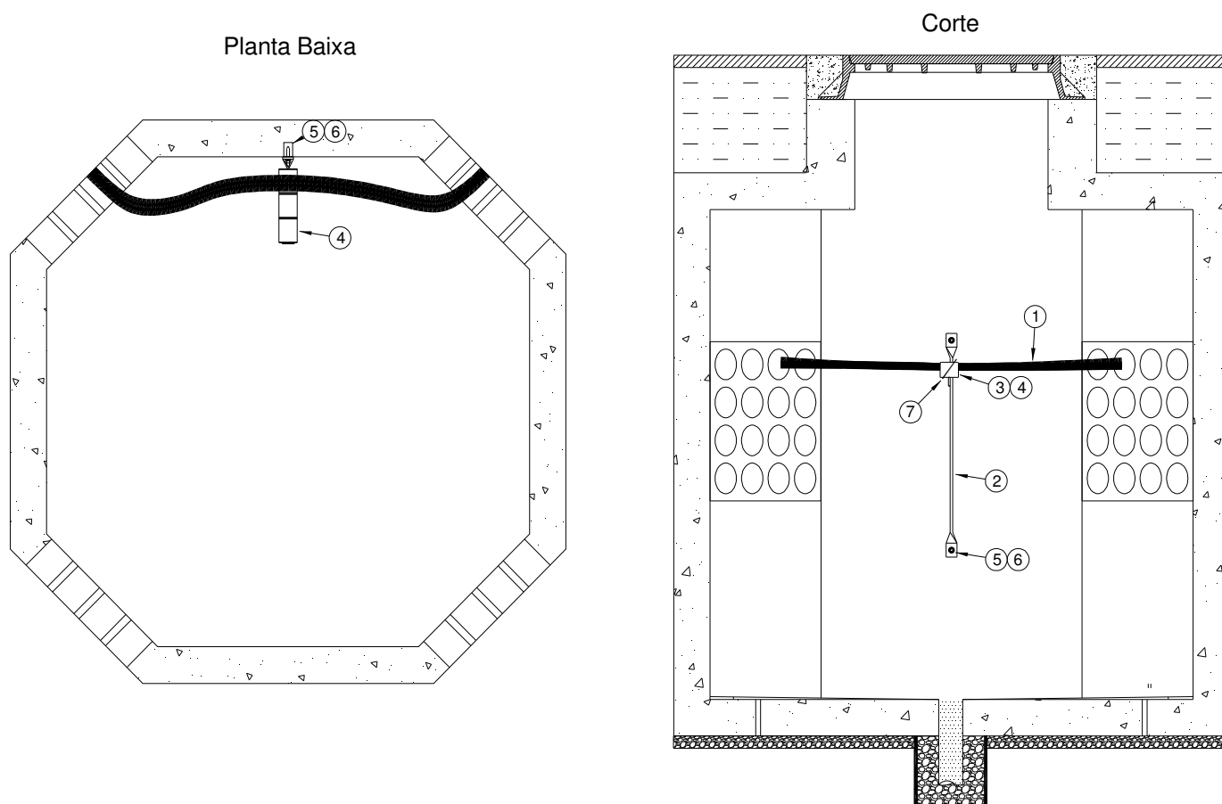
Figura 36 - Instalação de cabo em caixa M
