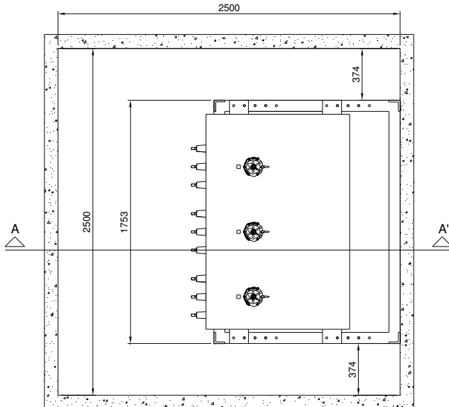
Planta Baixa
