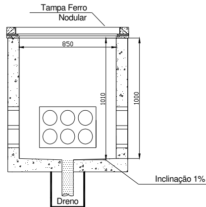
Corte BB'
