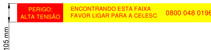
Figura 1 – Faixa de Sinalização e Advertência
