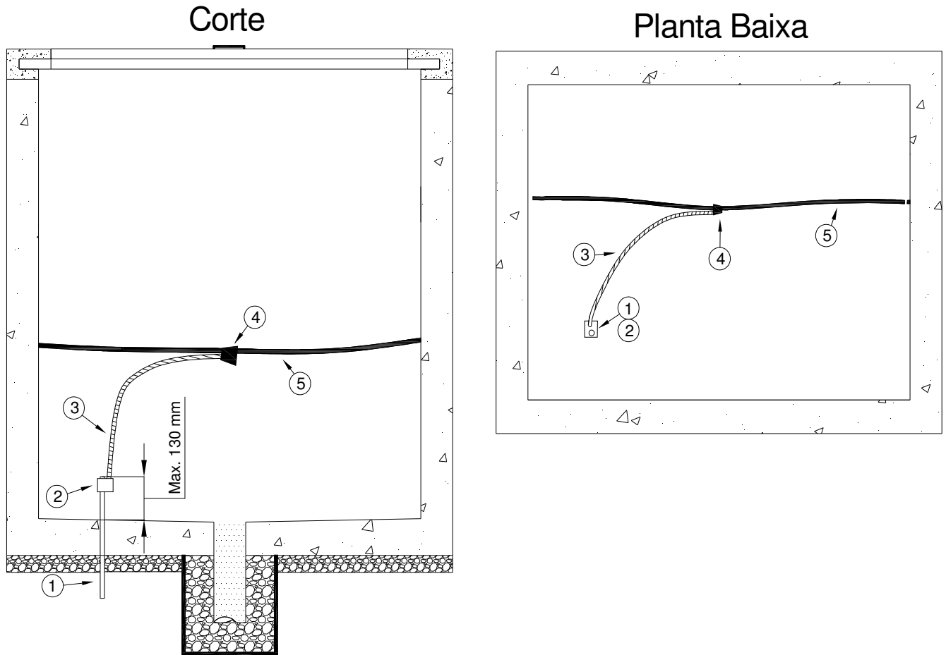
Figura 56- Instalação de Aterramento e Ligação ao Condutor de Proteção em Caixas Tipo D e E
