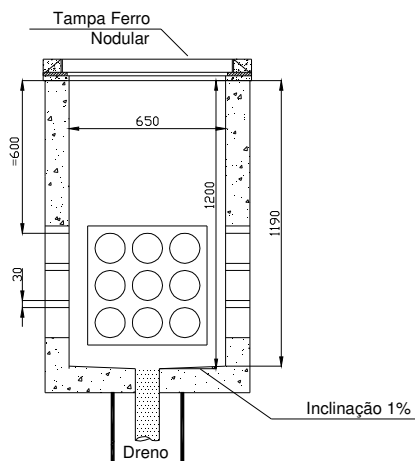
Corte AA'
