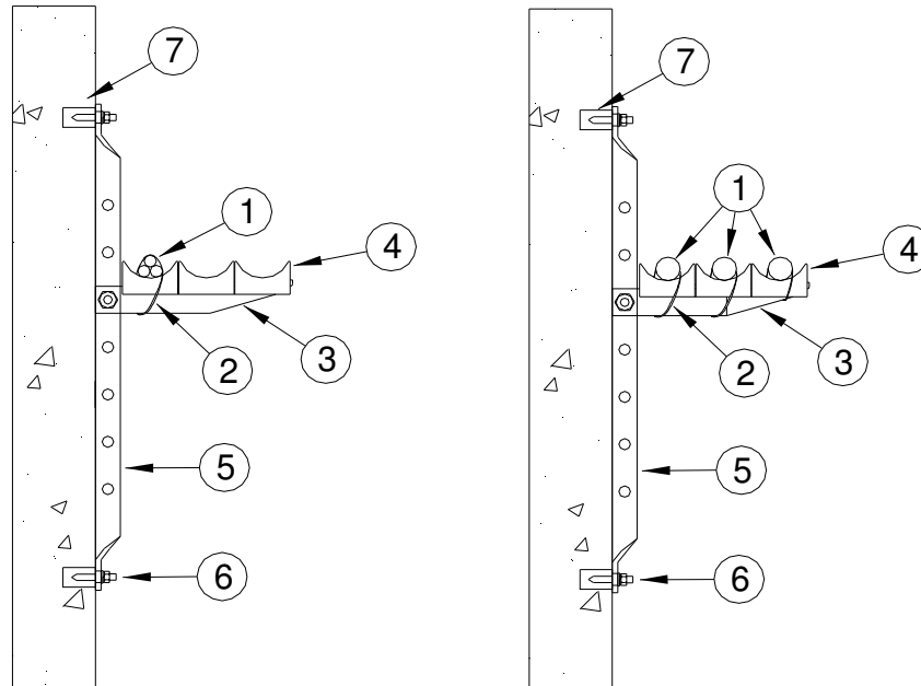
Figura 38 – Montagem de Suportes para Cabos e Desconectáveis em Caixas
