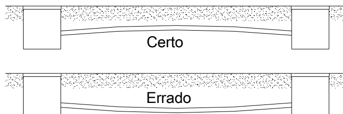
Figura 2 – Declividade em bancos de dutos
