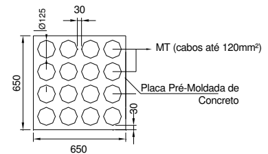
Placa Entrada/Saída Dutos
