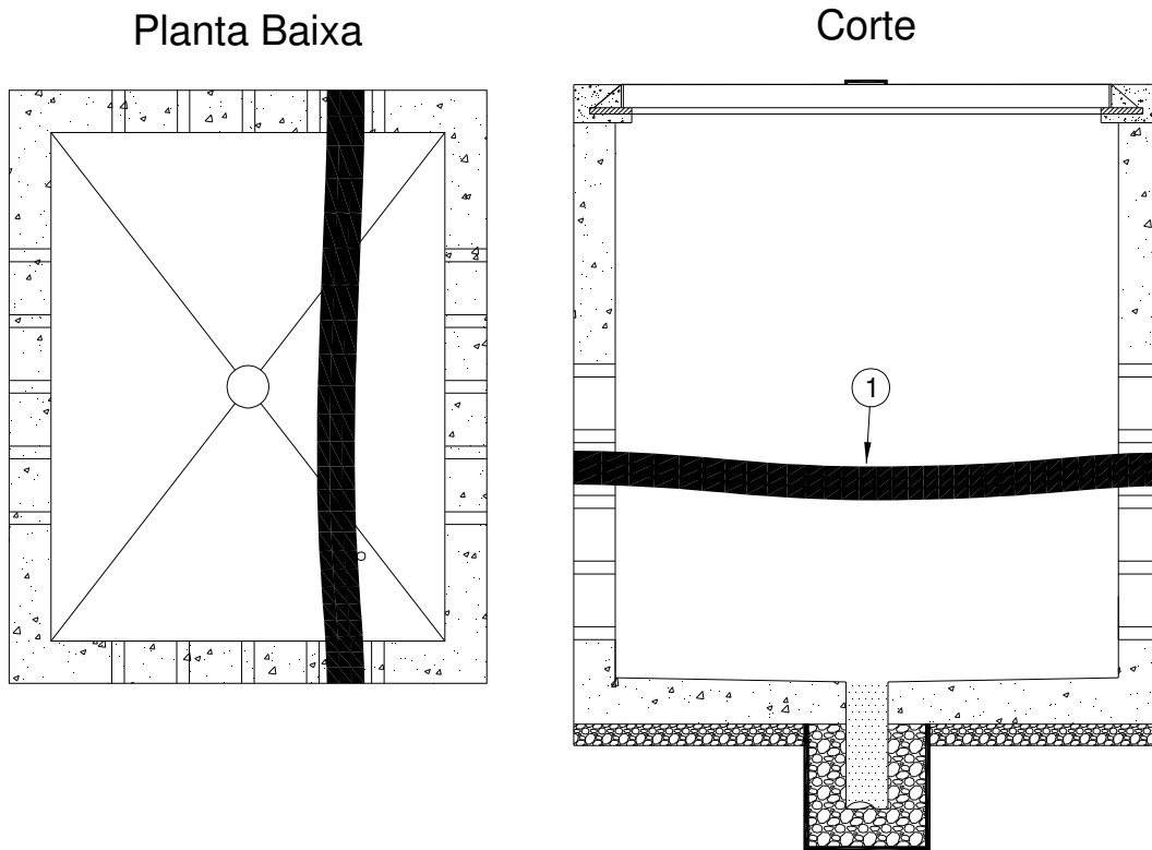
Figura 34 - Instalação de cabo em caixas D e E
