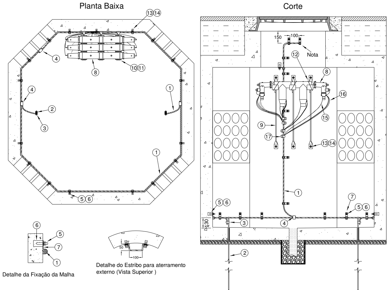
Figura 62 – Instalação de Aterramento e Ligação aos Desconectáveis 600A em Caixas Tipo M
