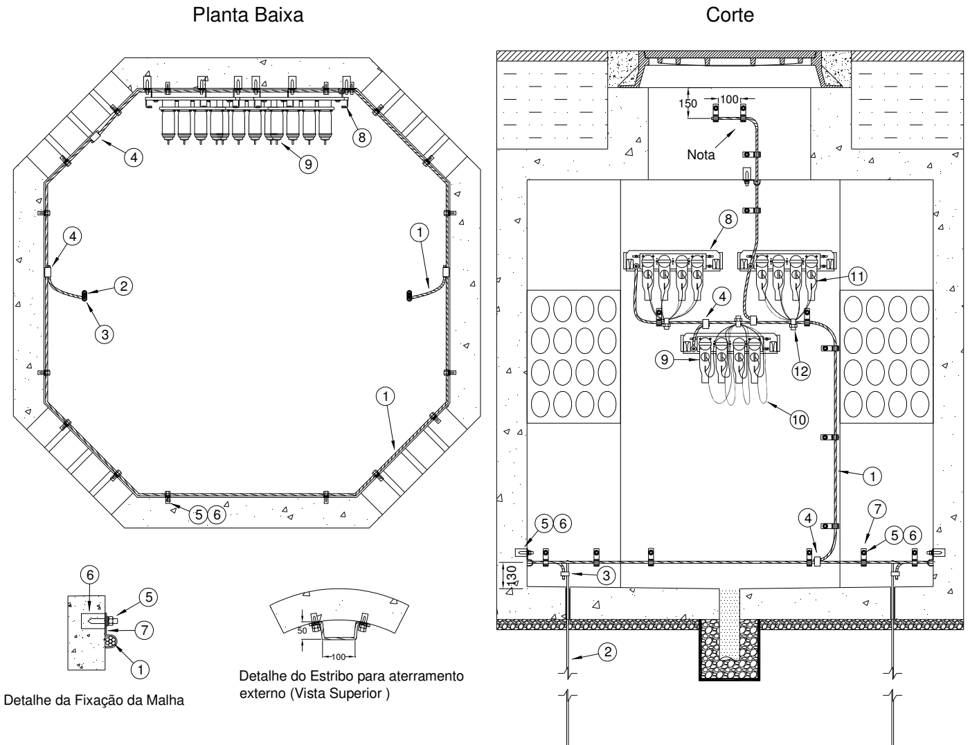
Figura 61 – Instalação de Aterramento e Ligação aos Barramentos Desconectáveis em Caixas Tipo M
