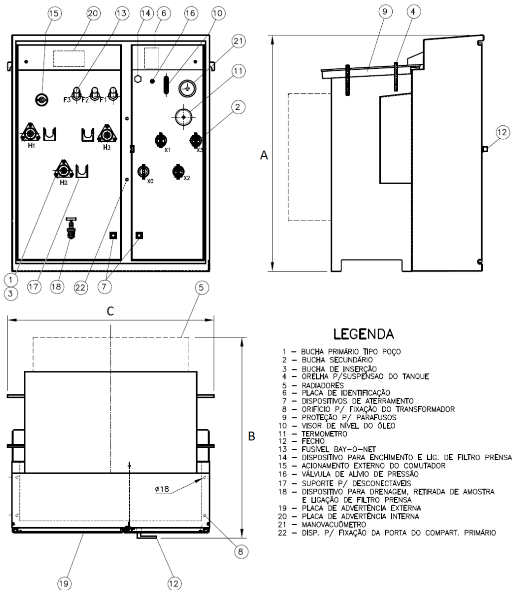
Características Dimensionais
