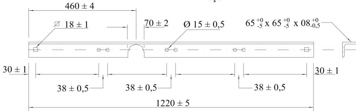
Peça 1
