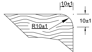
D etalhe 2
