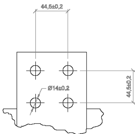
Terminal de BT, padrão NEMA, 4 furcos
