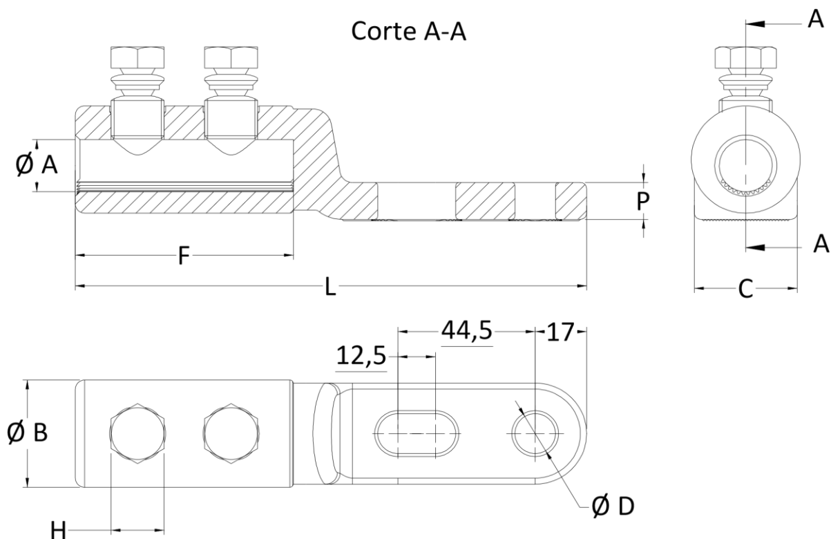
Terminal Torquimétrico 02 Furos NEMA para Condutores de Cobre e Alumínio Compactado
