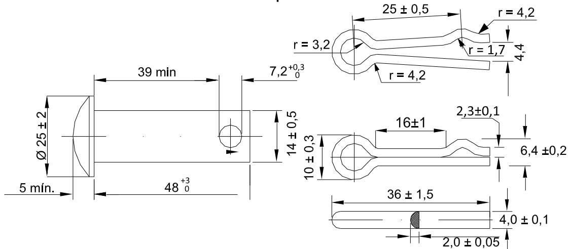
Detalhe: Pino e Cupilha
