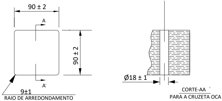
DETALHE PARA ENSAIO DE FLEXÃO
