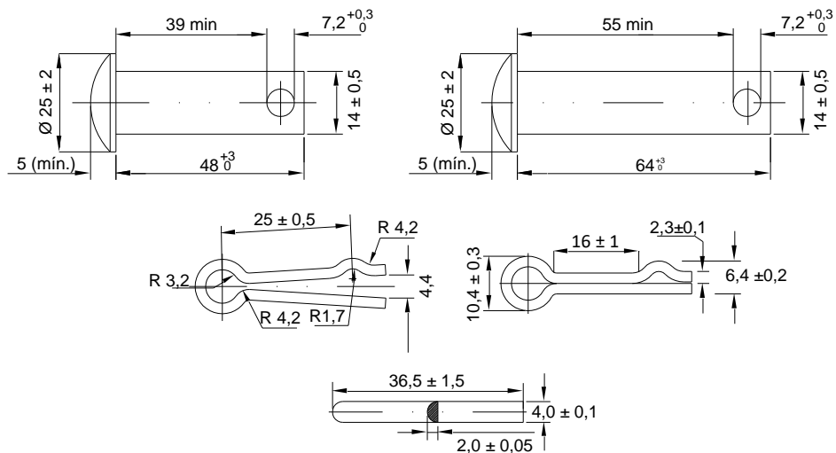
Detalhe: Pinos e Cupilha
