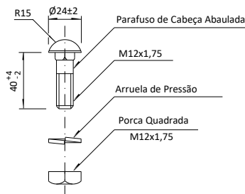
PEÇA - 2
