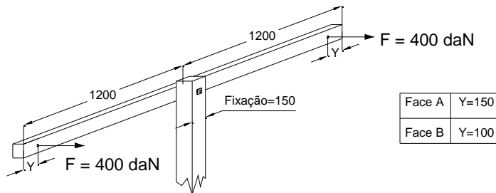
Detalhe para Ensaio de Flexão
