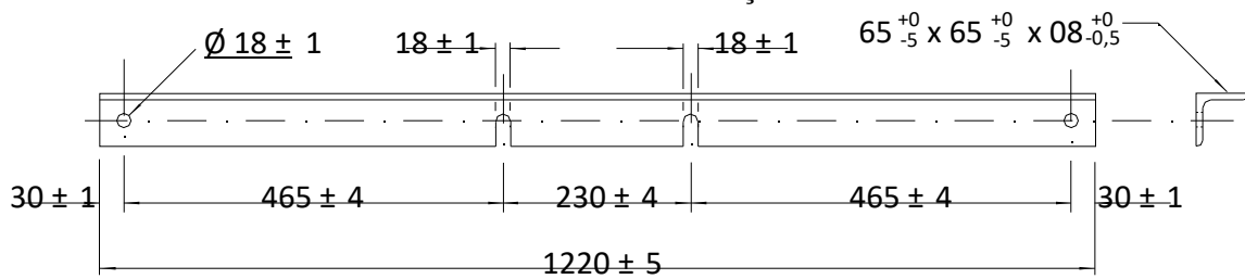
Peça 2
