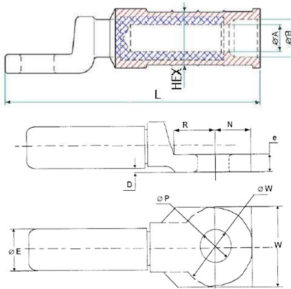
Dimensões para terminais pré-isolados
