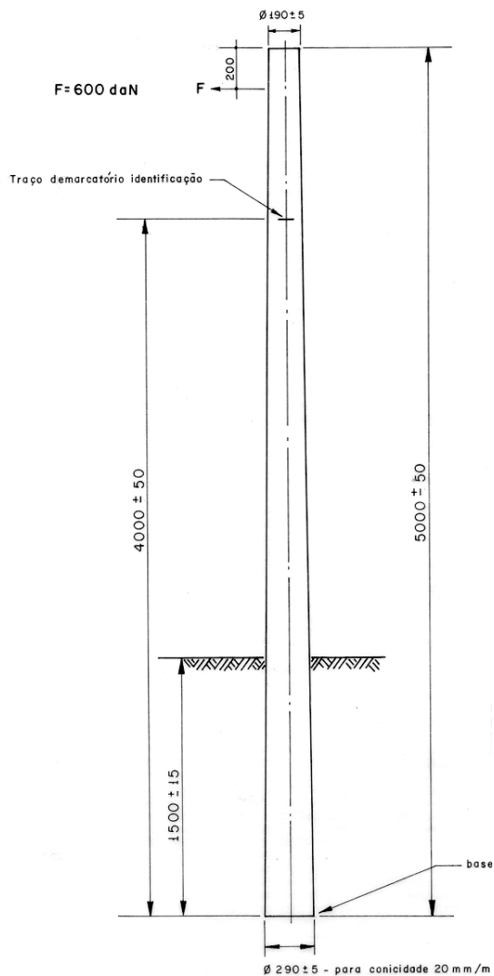
S-01 CONTRA-POSTE DE CONCRETO DE SEÇÃO CIRCULAR
