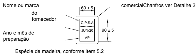
Detalhe 1
