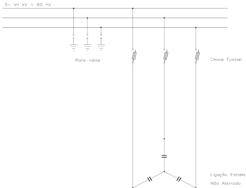
Diagrama Trifilar – Banco de Capacitores – Fixo
