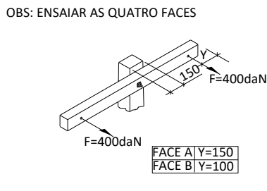
DETALHE PARA ENSAIO DE FLEXÃO
