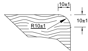
Detalhe 2
