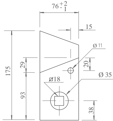
CUPILHA
