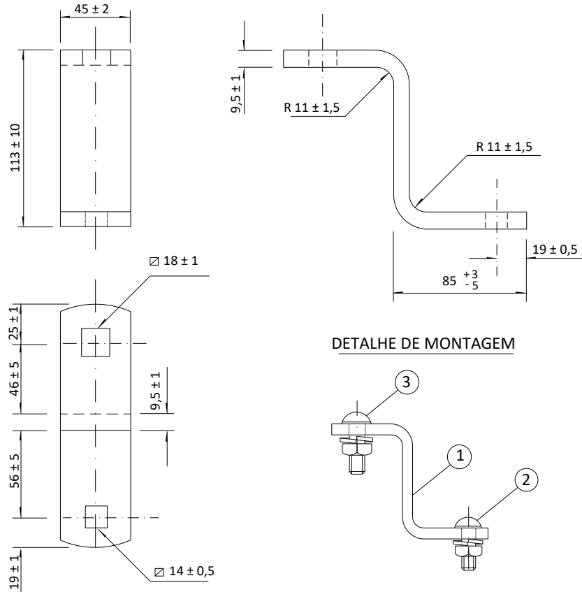
PEÇA - 1
