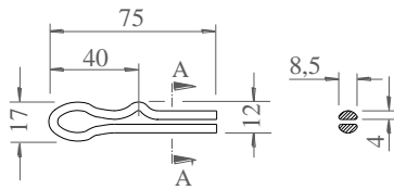
CUPILHA
