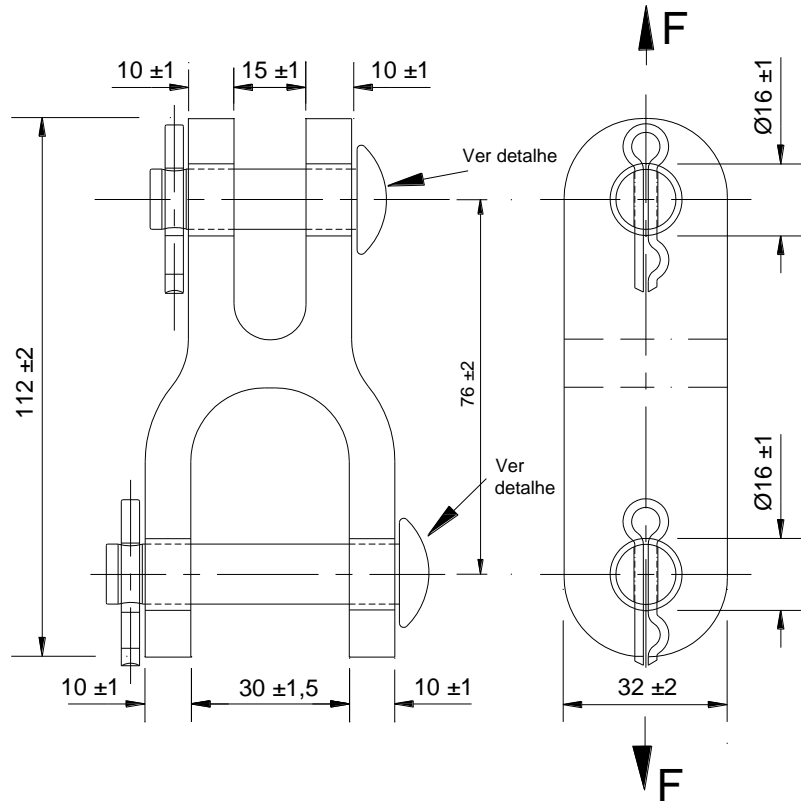
Detalhe: Pinos e Cupilha
