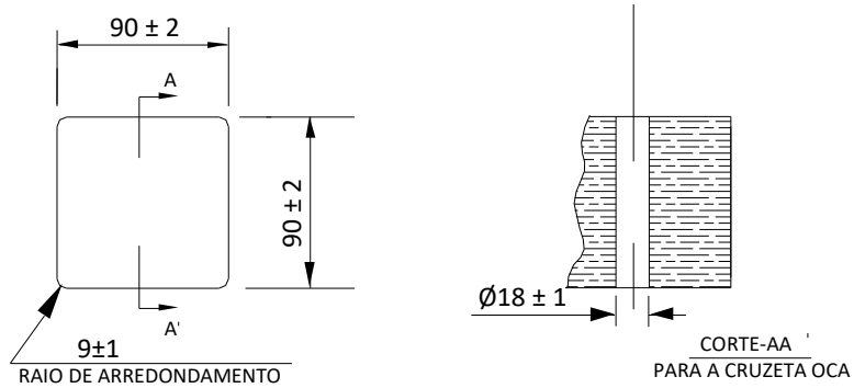
DETALHE PARA ENSAIO DE FLEXÃO
