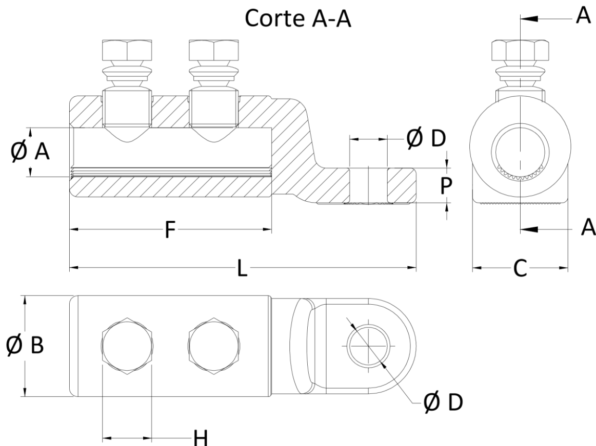
Terminal Torquimétrico 01 Furo NEMA para Condutores de Cobre e Alumínio Compactado
