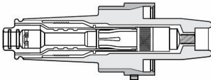
Terminal Desconectável Cotovelo 25 kV
