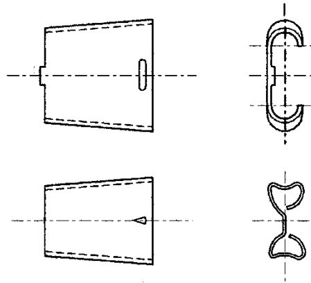
DESENHO ORIENTATIVO
