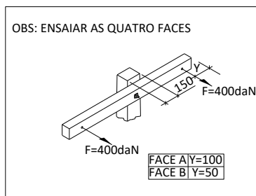
DETALHE PARA ENSAIO DE FLEXÃO
