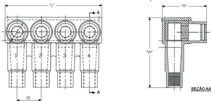
Alternativa 02 – Barramento Múltiplo Isolado
