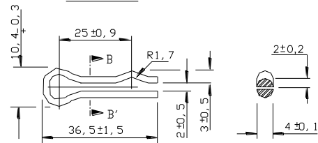
CUPILHA
