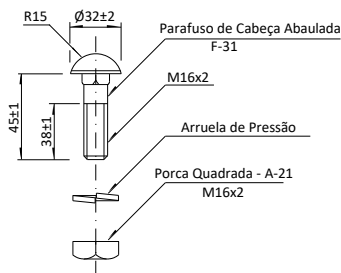
PEÇA - 3
